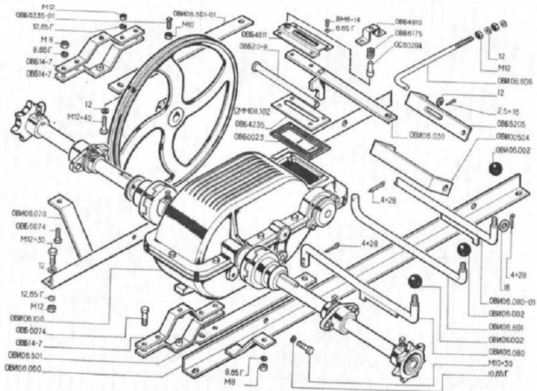
Рис. 28. Механизм самопередвижения ОВИ 06.000.
